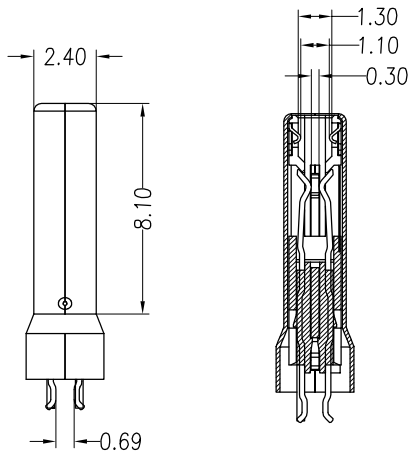
剖面 A-A 比例 1 : 1
