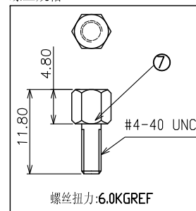
螺丝规格
